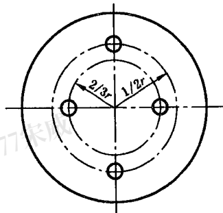
图 B.2 压痕位置
